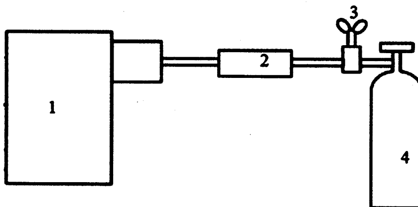
Рисунок В.1 – Рекомендуемая схема подачи ГС на вход газосигнализаторов 1 – газосигнализатор; 2 – ротаметр (индикатор расхода), 3 – редуктор; 4 – источник ГС (баллон или генератор газовых смесей)
